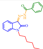
BZO-HEXOXIZID
