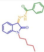
BZO-POXIZID
